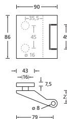
Glass door hinge pair Glass door hinge 3-part
